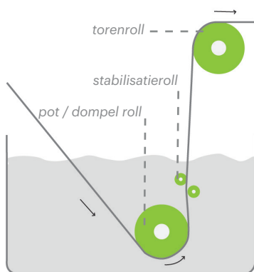
Schema van een zinklegering smeltbad (zinkbad)
